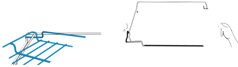
Figura 5: Desmontaje
